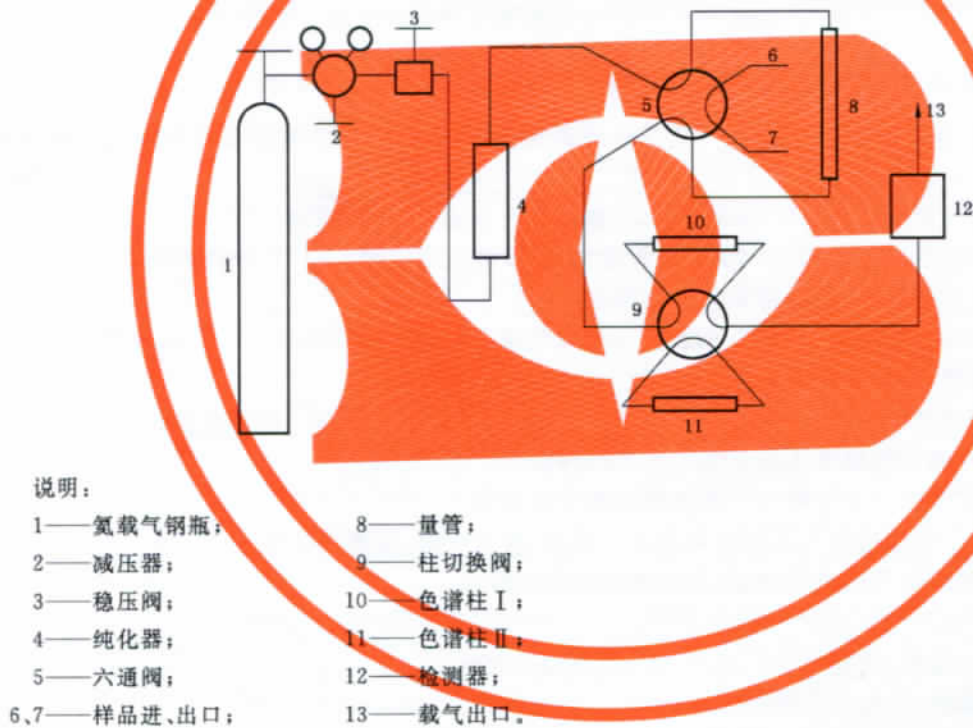
图 A.1 色谱流程图
